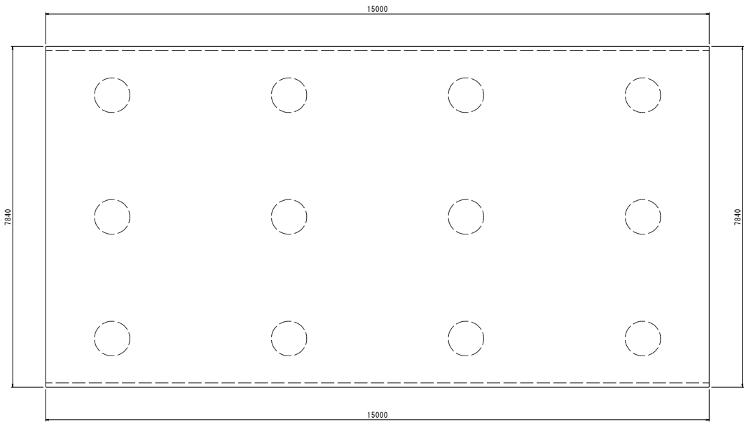
基礎伏図
