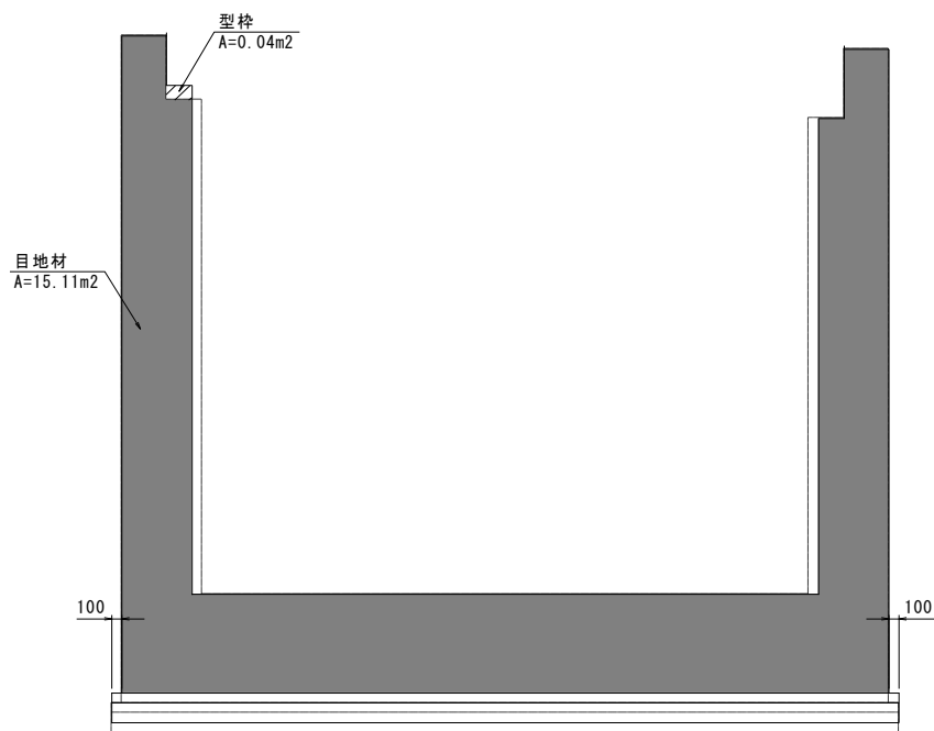
終点側 端部
