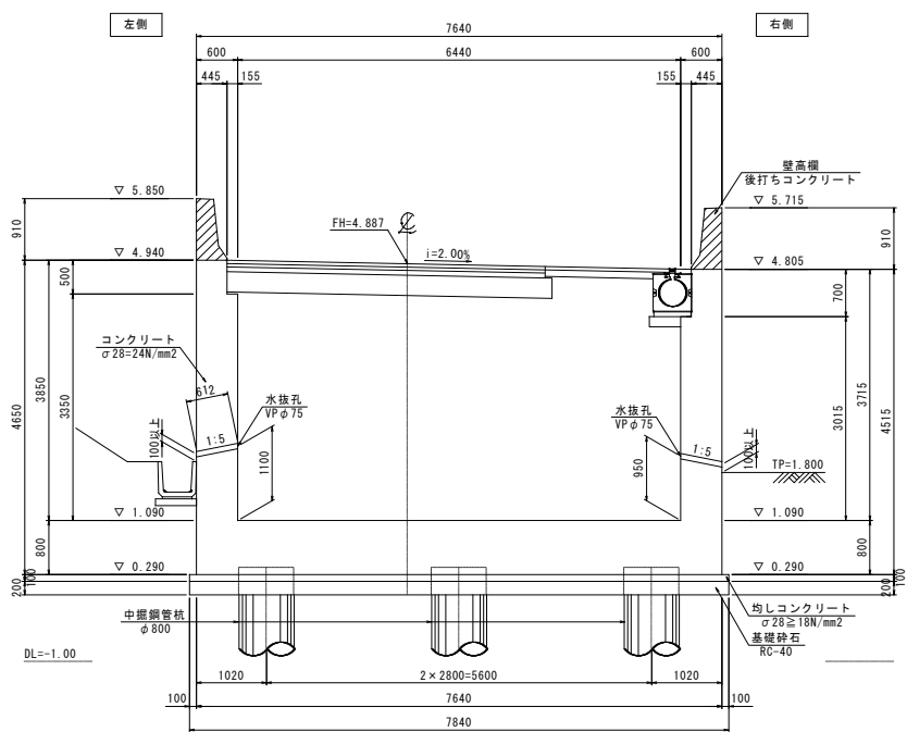
1-1断面
