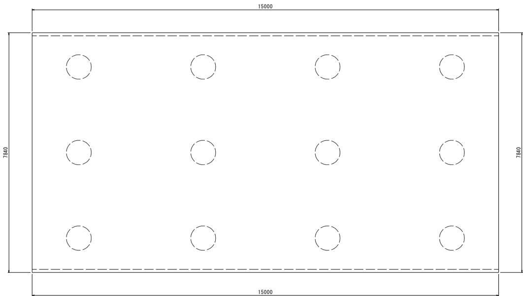
基礎伏図
