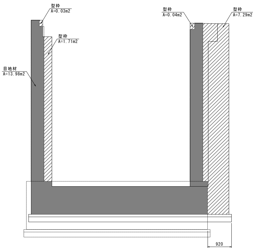
起点側 端部
