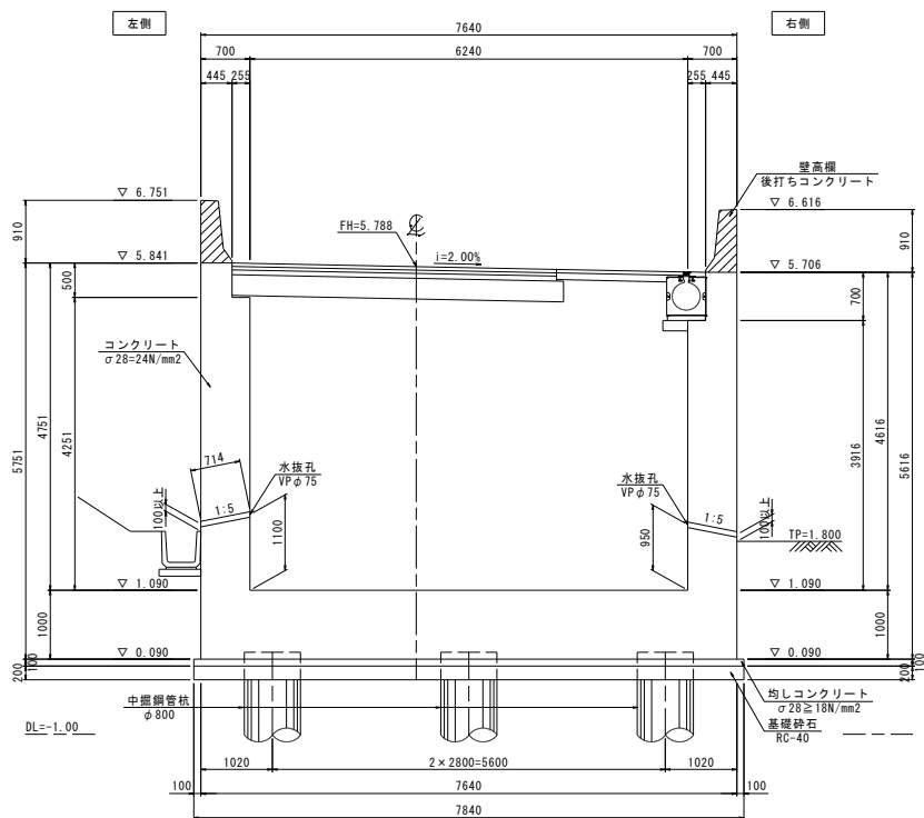
1-1断面
