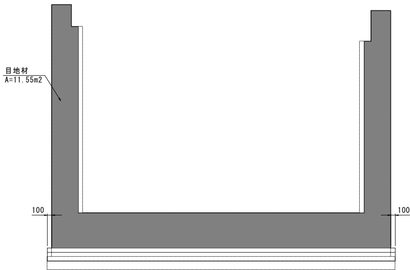
終点側 端部
